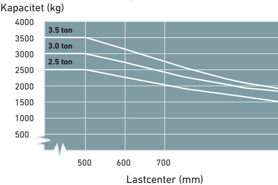
Kapaciteter ved forskellige lastcentre Simplex - h3 = 3300 mm
